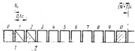
1—секундный маркер; 2—информационные сигналы
