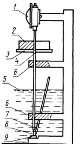
Схема прибора для испытания по Вика
