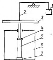
1—противовес; 2—проволока; 3—инерционная дельта; 4—верхний подвижный зажим; 5—образец; 6—термостатирующая камера; 7—нижний неподвижный зажим
