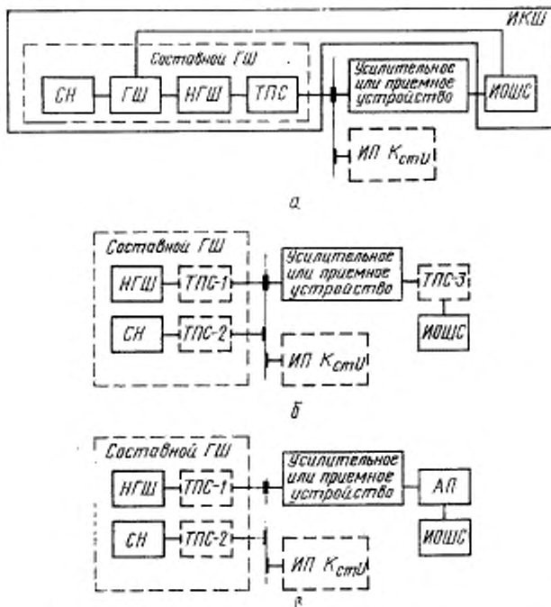
а—схема стенда для измерения ЭШТВ устройств с использованием НГШ проходного типа и ИКС в автоматическом режиме; б—то же, с использованием НГШ непроходного типа; в—схема стенда для прецизионных измерений
