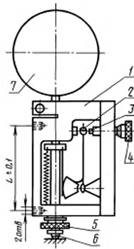
1 — корпус; 2 — подвижные контак- ты; 3 — неподвижные контакты; 4 — настроочный винт; 5 — микровинт по- дачи; 6 — измерительный наконеч- ник; 7 — отчетное устройство
