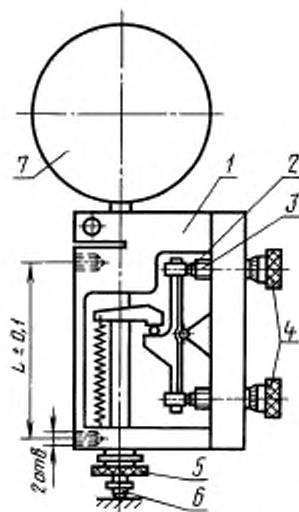
1 — корпус; 2 — подвижные контакты; 3 — неподвижные контакты; 4 — на- строочные винты; 5 — микровинт пода- чи; 6 — измерительный наконечник; 7 — отче- тное устройство
