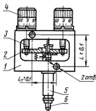
1 — корпус; 2 — подвижный контакт; 3 — неподвижные контакты; 4 — на- строочный винт; 5 — гильза; 6 — из- мерительный наконечник
