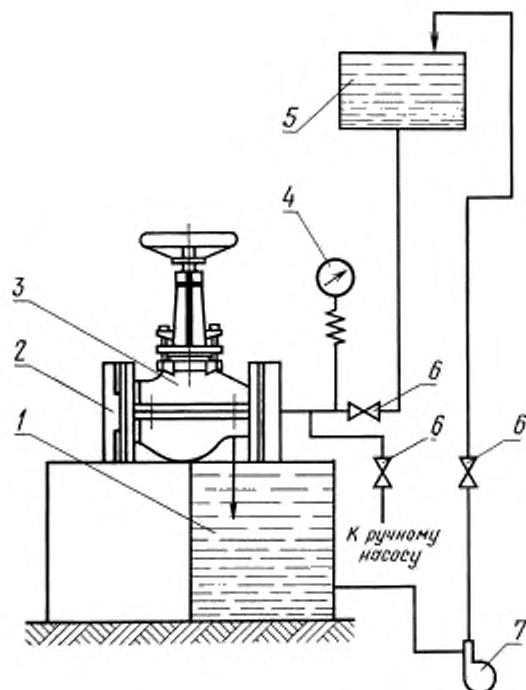
1 — емкость для слива воды; 2 — подвижный зажим; 3 — испытываемое изделие; 4 — манометр; 5 — емкость для воды; 6 — запорный пентиль; 7 — центробежный насос
