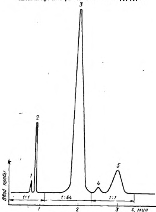
Типовая хроматограмма технического фурфурола
