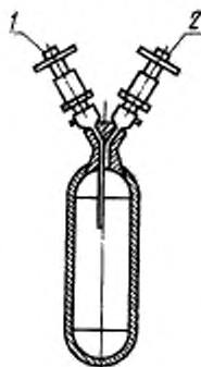
1, 2 — вентили Черт. 1
