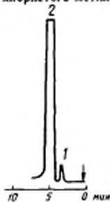
Хроматограмма искусственной смеси диметилового эфира и хлористого метила
