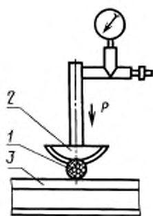
1 — испытуемый образец; 2 и 3 — матрицы
