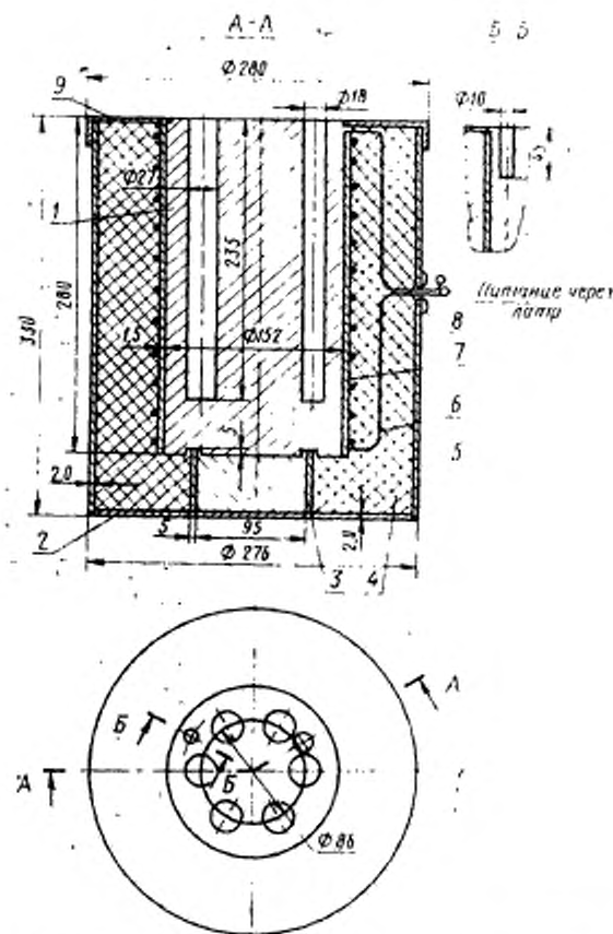
1—корпус блока; 2—дно; 3—пластина опорная; 4—изоляция; 5—кожух; 6—провод; 7—трубка; 8—трубка фарфоровая; 9—крышка
