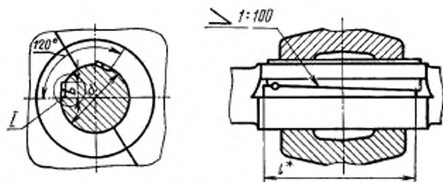
Размеры сечений шпонки и шпоночного паза.
