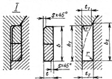
Размеры сечений шпонки и шпоночного паза.
