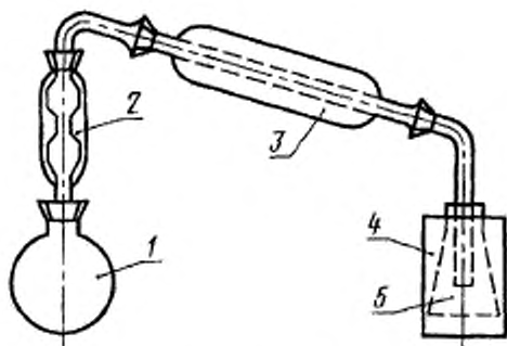
1 — круглодонная колба; 2 — изгиб; 3 — холодильник; 4 — вилонж; 5 — цилиндр
