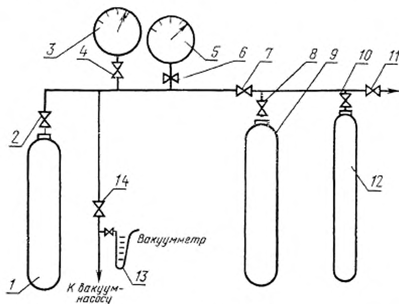
1, 9, 12—баллоны; 3, 5—манометры; 2, 4, 6, 7, 8, 10, 11, 14—вентили; 13—вакуумметр
