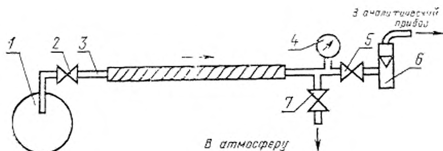
1—заводской трубопровод; 2, 5, 7—клапаны; 3—трубопровод для подачи газа к месту анализа; 4—манометр; 6—ротаметр, реометр или другой газовый счетчик
