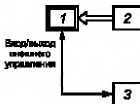
1 — испытываемое оборудование станции радиоконтроля; 2 — генератор стандартных сигналов, 3 — внешний компьютер
