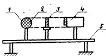
1 — изотопный источник быстрых нейтронов; 2 — шаровый замедлитель; 3 — кадмиевый экран; 4 — блок детектирования; 5 — градуировочная линейка
