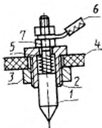
Схема зонда
