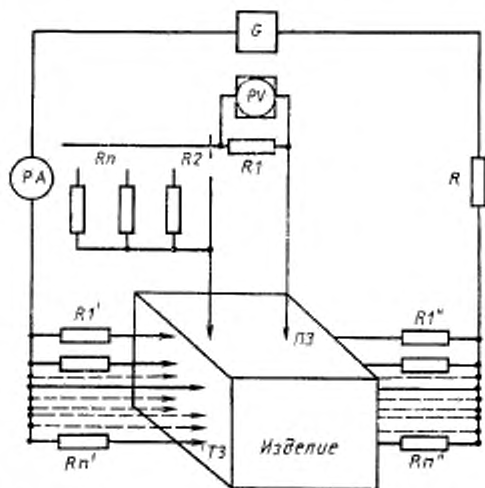
G — источник постоянного тока; PA — прибор для измерения тока; PV — прибор для измерения напряжения; R — ограничивающий резистор; P_1 - R_n — резисторы делителя напряжения; R_1' - R_n' , R_1'' - R_n'' — добавочные резисторы; T_3 — токовый зонд; ПЗ — потенциальный зонд
