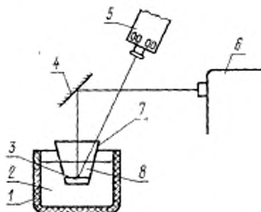
1—платиновая чашка; 2—жидкий азот; 3—анализуемый раствор; 4—зеркало; 5—осветитель; 6—монокроматор; 7—платиновый тигель; 8—жидкий азот.
