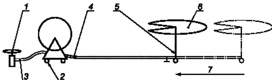
1 — источник воды; 2 — стационарный барабан; 3 — труба/шланг от источника воды; 4 — раздаточная труба (тянущего типа); 5 — тележка; 6 — устройство или система распределения воды: дождевальная машина, в том числе пушечного типа, штанга (на тележке); 7 — направление движения
