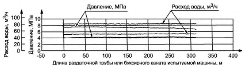
е) Отклонения давления и расхода воды
