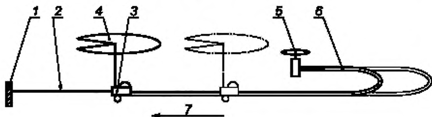
1 — якорь буксирного каната; 2 — буксирный канат; 3 — тележка; 4 — устройство или система распределения воды: дождевальная машина, в том числе пушечного типа, штанга (на тележке); 5 — источник воды; 6 — раздаточный шланг; 7 — направление движения
