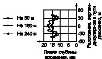
b) Глубина орошения зон перекрытия на выбранных поперечных линиях
