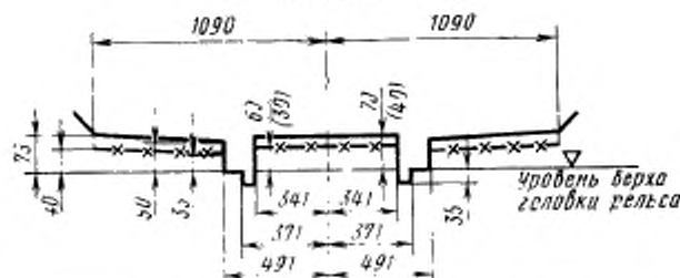
Нижнее очертание габарита
