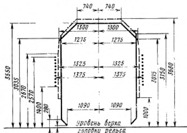
ГАБАРИТ Tu Верхнее очертание габарита
