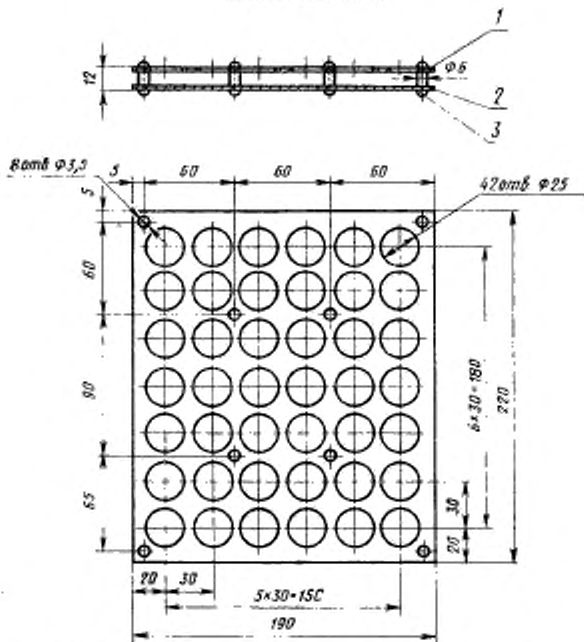
1—фиксатор тиглей; 2—основание; 3—соединительная стойка.
