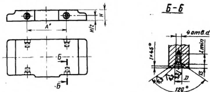
Размеры, мм
