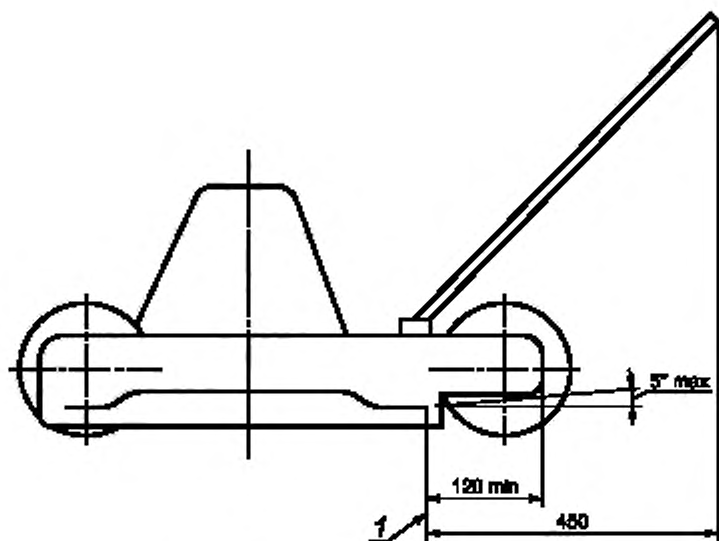
Рисунок 101 — Безопасные расстояния для ротационных приборов
