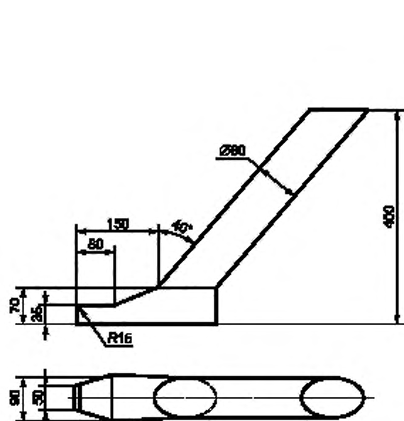
Рисунок 103 — Имитатор стопы
