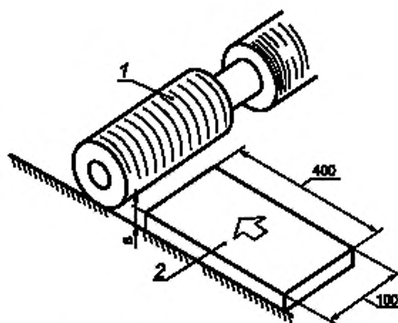
Рисунок 105 — Прочность режущего устройства
