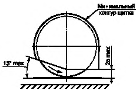
Рисунок 108 — Ограждение режущих устройств сбоку
