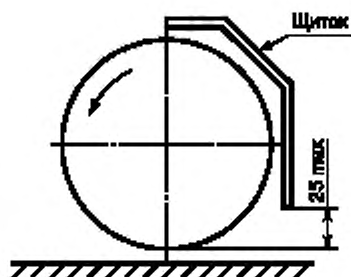
Рисунок 110 — Ограждение передних разгрузочных проемов
