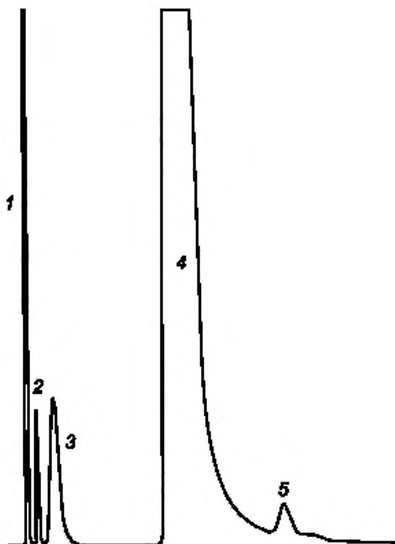
1 — диэтиловый эфир; 2 — n -октан — «внутренний эталон»; 3 — уксусный альдегид; 4 — этиловый спирт; 5 — кротоновый альдегид
