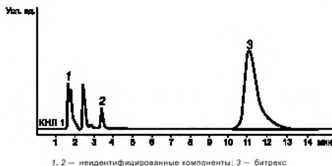
Рисунок 2 — Типовая хроматограмма градуировочного раствора
