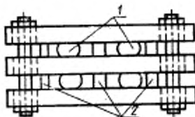
1—образцы, 2—ограничители
