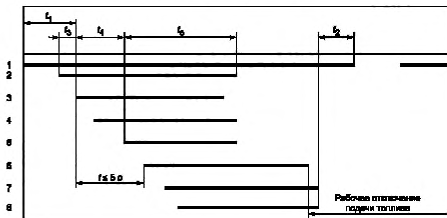
Диаграмма нормальной работы горелки
