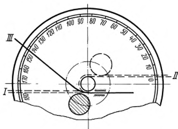
Схема испытания ленты на пружинность
