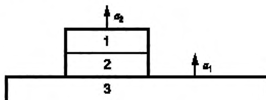
1 — масса нагрузки m ; 2 — упругий материал; 3 — вибровозбудитель
