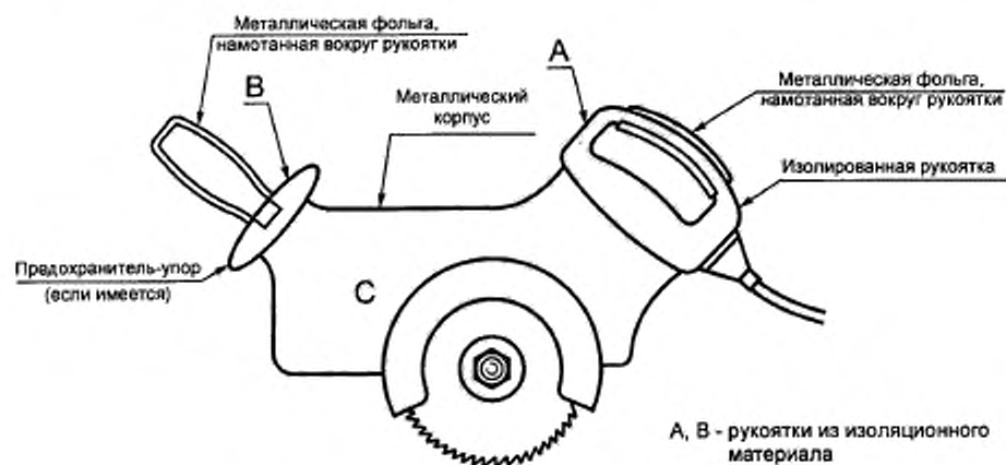
Рисунок 8в — Ручная (портативная) электропила
