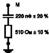
Рисунок 8а — Элемент RC
