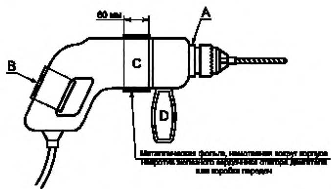
Рисунок 8б — Ручная (портативная) электрическая дрель
