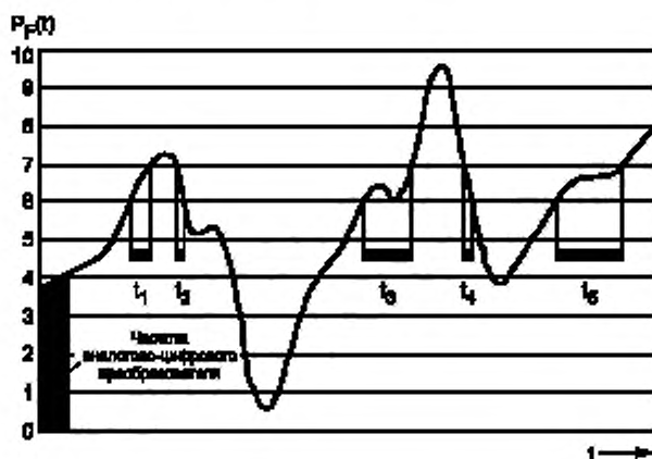
Рисунок 2а — Уровень фликера как функция времени
