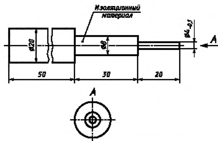
Рисунок Г.3 — Стандартный испытательный штырь
