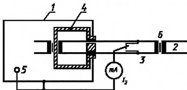
Рисунок Ж.1 — Схема для измерения силы тока утечки аппаратов группы II.1
