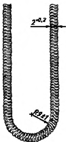
Рисунок Г.4 — Испытательная цепочка
