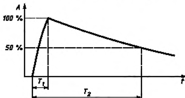
Рисунок Е.1 — Схема для испытания импульсным перенапряжением
