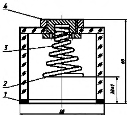
1 — прокладки; 2 — пластина; 3 — пружина; 4 — контакт
