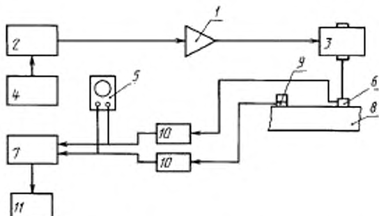
1 — усилитель мощности, 2 — устройство регулировки амплитуды, 3 — виброисполнитель, 4 — генератор сигналов, 5 — контрольный осциллограф, 6 — преобразователь сил, 7 — анализатор, 8 — испытуемая конструкция, 9 — преобразователь вибрации, 10 — форматор сигнала, 11 — графопроектор для другой выходной прибор
