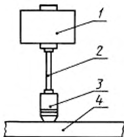
1 — виброизбудатель, 2 — толкатель, 3 — импедансная головка 4 — испытуемая конструкция
