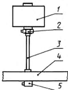
1 — виброисполнитель, 2 — преобразователь силы, 3 — плавитель; 4 — испытуемая конструкция; 5 — акселерометр
