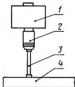
1 — виброисполнитель, 2 — измеренная плочка; 3 — плавитель; 4 — испытуемая конструкция
