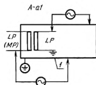
1 — ДОСТУПНАЯ МЕТАЛЛИЧЕСКАЯ ЧАСТЬ
