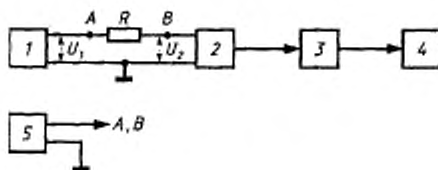
1 — генератор сигналов НЧ по 6.2.8; 2 — передатчик; 3 — элемент антенны по 6.2.3; 4 — девиометр по 6.2.9; 5 — вольтметр НЧ по 6.2.10; R — измерительное сопротивление 600 Ом \pm 0,5 %
