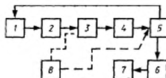
1 — анализатор боковых полос по 6.2.2; 2 — передатчик; 3 — согласованная нагрузка по 6.2.3; 4 — аттенуатор дополнительный; 5 — согласованный трюнк; 6 — демодулятор по 6.2.1; 7 — осциллограф по 6.2.6; 8 — направленный ответвитель по 6.2.4
