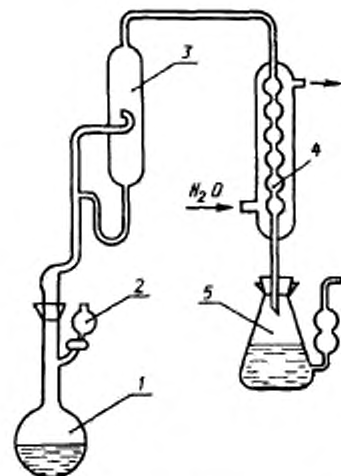
1 — колба стеклянная круглодонная; 2 — воронка стеклянная каплевая; 3 — каплеуловитель; 4 — холодильник стеклянный шариковый; 5 — колба коническая
