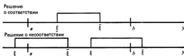
Рисунок 2 — Правила принятия решений при контроле поставщика по методу толерантных границ
