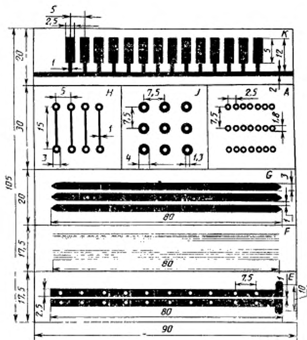
Рисунок 1 — Составной рисунок для испытаний
