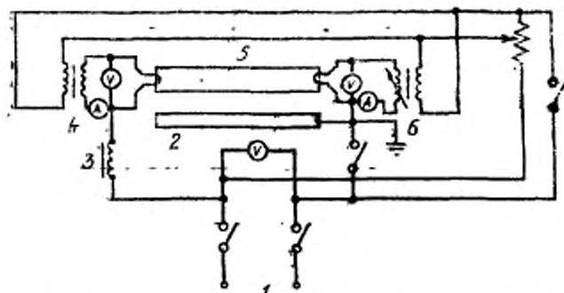
1 — источник питания; 2 — зажигающая полоса; 3 — балласт; 4, 5 — трансформаторы; 6 — лампа
