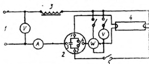
1 — источник питания; 2 — стартер; 3 — образцовый балласт; 4 — лампа; 5 — дополнительный выключатель
