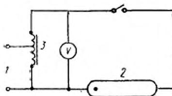
1 — источник питания; 2 — лампа; 3 — балласт
