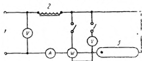
1 — источник питания, 2 — образцовый балласт; 3 — лампа;
