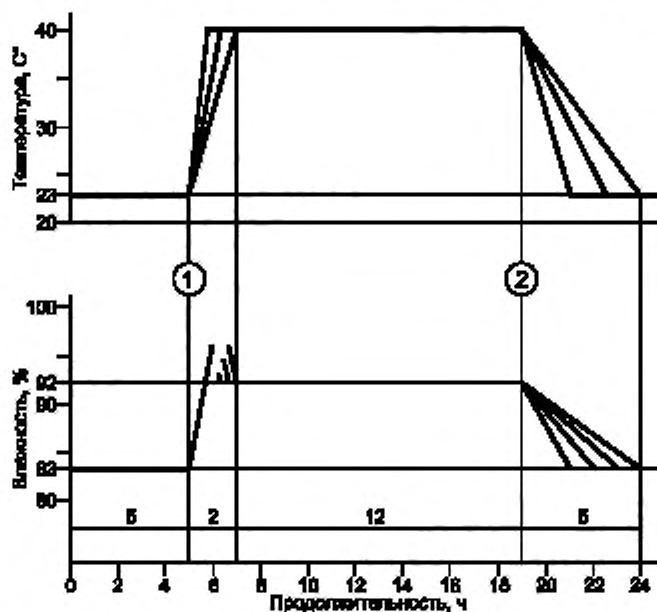
Рисунок 2 — Изменения температуры и влажности по циклам
