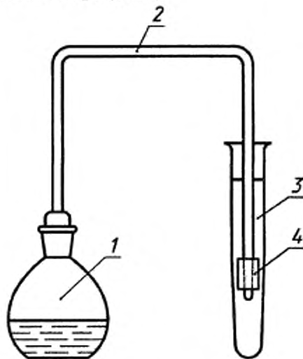
1 — колба плоскодонная со шлифом вместимостью 50—100 см 3 , 2 — трубка П-образная изогнутая диаметром 5 мм с оттянутым в капилляр концом, прикрепленная на шлифе к плоскодонной колбе 1. 3 — сосуд поглотительный — коническая пробирка вместимостью 10 см 3 ; 4 — трубка короткая стеклянная диаметром 6—7 мм
