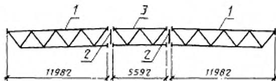
Ферма пролетом 30 м
