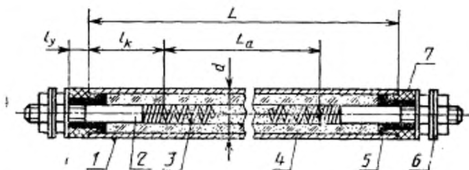
1—оболочка; 2—контактный стержень; 3—нагревательный элемент; 4—наполнитель; 5—герметизирующий материал; 6—контактные гайки и шайбы; 7—изолятор; L — развернутая длина трубки; L_a — активная длина; l_x — номинальная длина контактного стержня ТЭН в заделке; d — диаметр уплотненного ТЭН; l_y — длина пути утечки тока.
