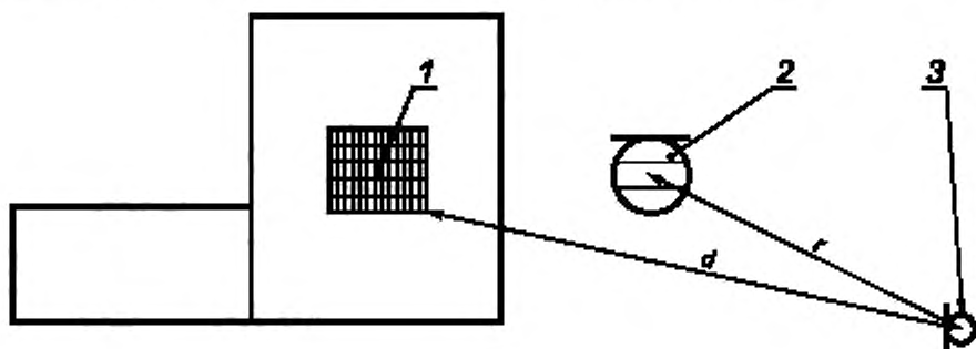
Рисунок В.6 — Положение микрофона относительно различных источников шума при виде сверху
