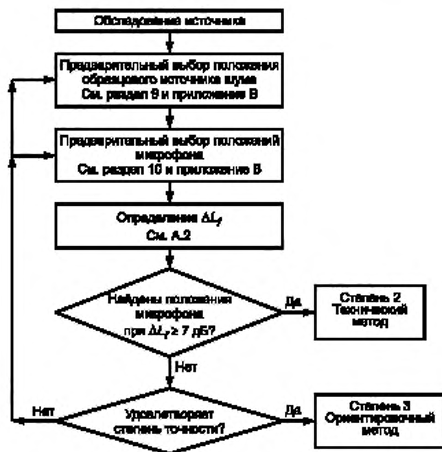
Рисунок А.1 — Схема действий для определения показателя реверберационности поля и достигаемой степени точности
