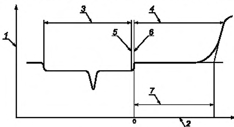
Рисунок В.2 — Определение ВОИ по термограмме
