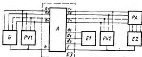
G —источник постоянного напряжения; PV1 —измеритель постоянного напряжения; A —НСН; a_1, a_2, \dots, a_n , b —входы НСН; c_1, c_2, \dots, c_n , f —выходы НСН; E1 —блок делителей; PV2 —измеритель постоянного напряжения; PA —измеритель постоянного тока; E2 —блок нагрузок НСН; E3 —устройство задания температурного режима; d_1, d_2, d_3 —выводы подключения обратной связи
