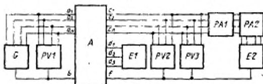
G —источник постоянного напряжения; PV1 , PV2 —измерители постоянного напряжения; A —НСН; a_1, a_2, \dots, a_N , b —входы НСН; c_1, c_2, \dots, c_N , f —выходы НСН; d_1, d_2, d_3 —выходы подключения обратной связи; E1 —блок делителей; PV3 —измеритель переменного (синусоидального, импульсного) напряжения; PA1 —измеритель постоянного тока; PA2 —измеритель переменного тока; E2 —блок нагрузок НСН
