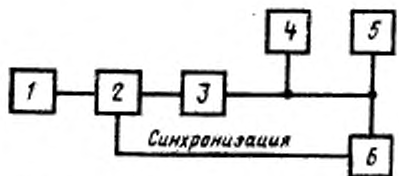
1 — генератор высокочастотных сигналов; 2 — прерыватель сигнала; 3 — приемник; 4 — вольтметр переменного тока; 5 — эквивалент нагрузки; 6 — осциллограф
