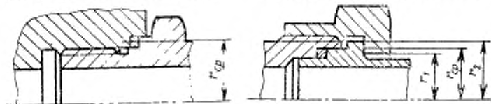
в) Фланцевое соединение
