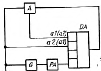
А — вспомогательное устройство балансировки (ВУБ); ДА — проверяемый ОУ или КН, G — источник постоянного напряжения, PA — измеритель постоянного тока, а — инвертирующий вход; а' — неинвертирующий вход.
