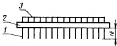
1—игольчатые электроды; 2—диск; 3—проводник
