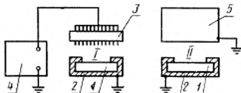
1 и II положение образца при электризации и измерения поверхностного заряда соответственно. 1—образец; 2—держатель образца; 3—коронирующий электрод; 4—источник высокого напряжения; 5—измеритель электростатического поля.
