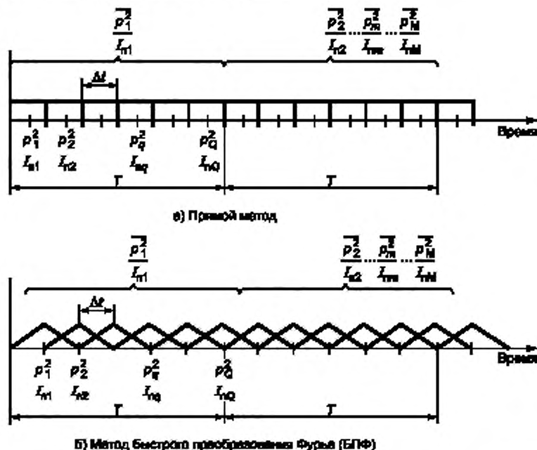
Рисунок 3 — Вычисление усредненных по времени интенсивностей звука \bar{I}_{nm} и квадратов звукового давления \bar{p}_m^2 , m = 1, 2, 3, \dots, M на времени усреднения T по измеренным последовательным значениям интенсивности I_{nQ} и квадрату звукового давления p_Q^2
